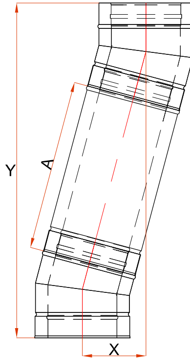
2 Coude 15°
