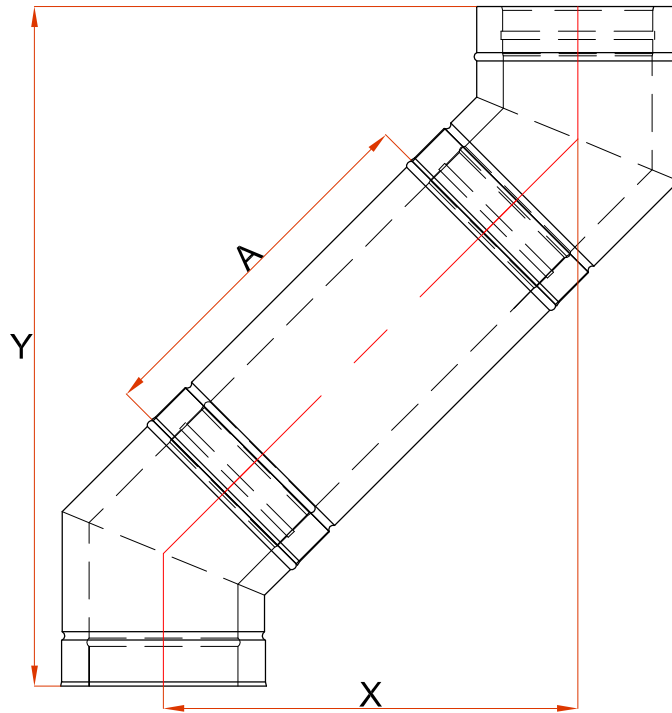
2 Coude 45°
